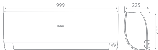
DIMENSÕES DE FIXAÇÃO
